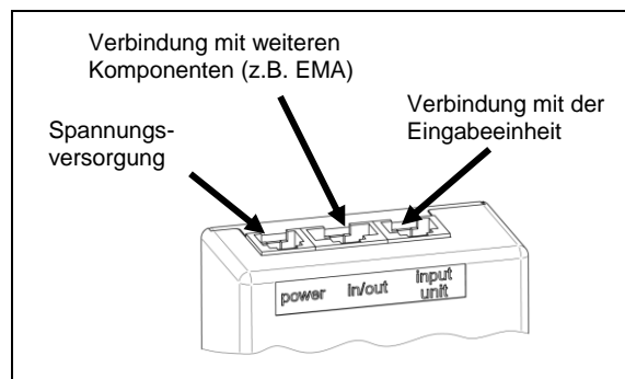
Abbildung 4: Anschlüsse am Schlossgehäuse
